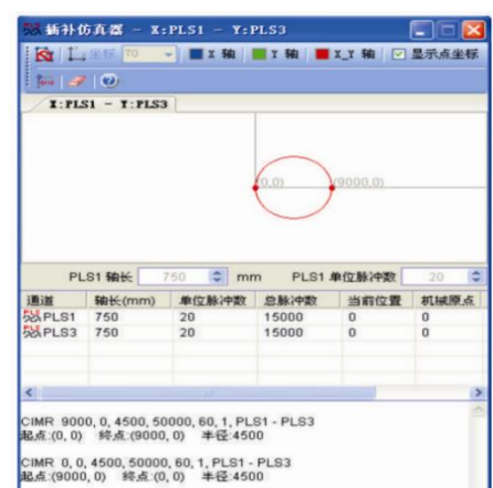
插补仿真器
